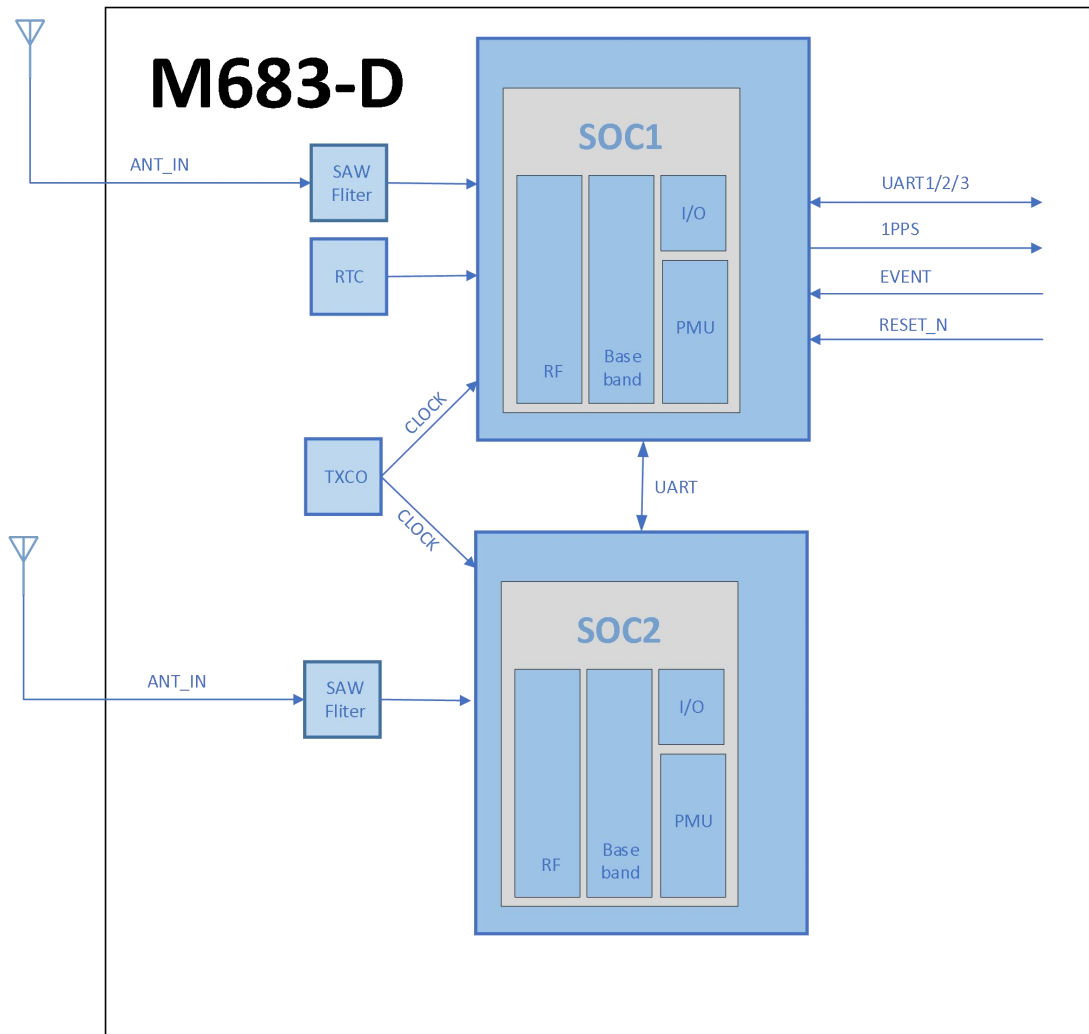
图 1-2 M683-D 系统框图
