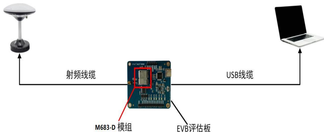
图 4-1 连接示意图
