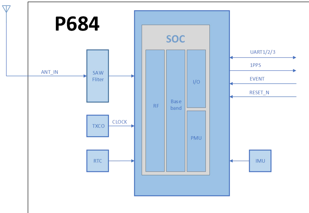
图 1-2 P684 系统框图
