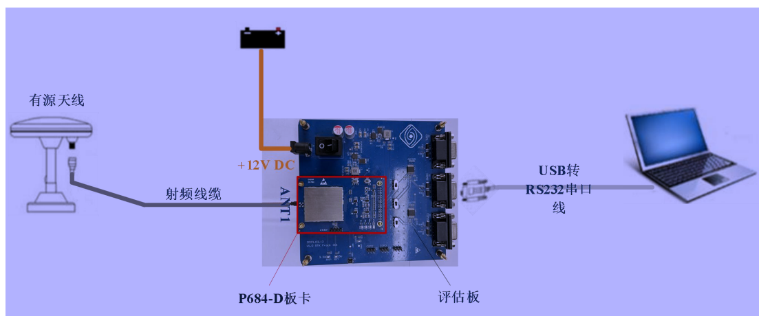
图 4-1 P684-D 连接示意图
